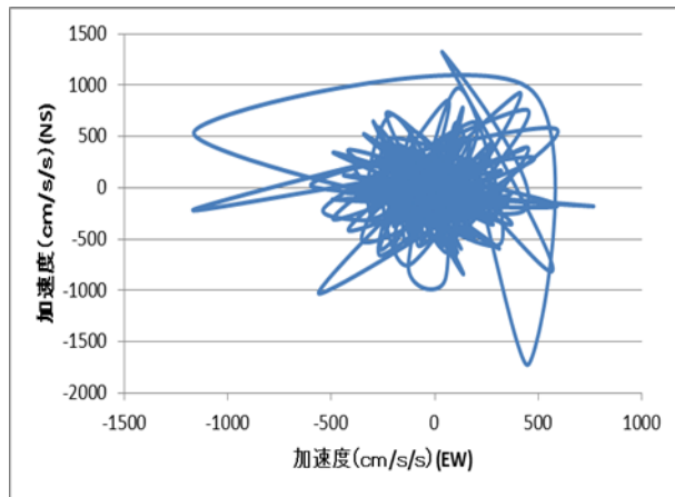
図2 東北地方太平洋沖地震のオービット（築館）
