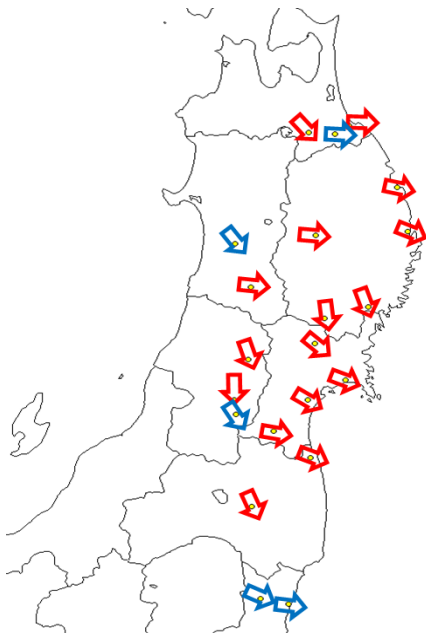
図3 東北地方太平洋沖地震の平均方向
