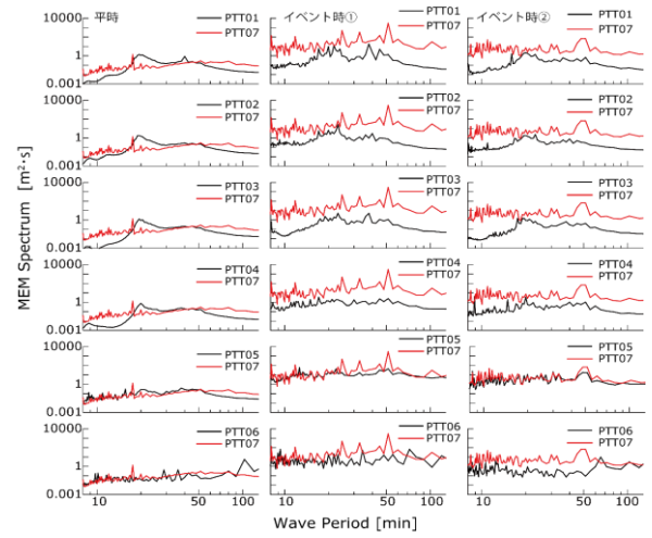
図-2 各観測点における MEM スペクトル
