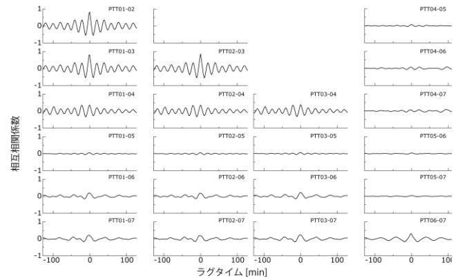
図-3 各観測点間における相互相関関数
