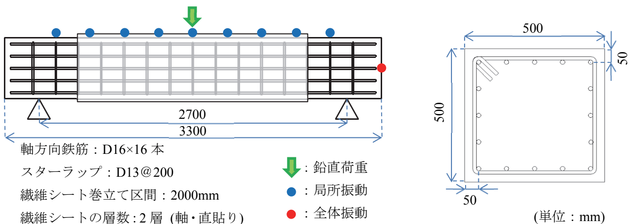
図-1 RC はり供試体概略図
