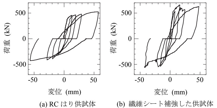
図－2 荷重－変位関係
