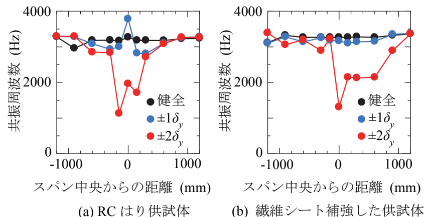
図－3 局所振動試験結果
