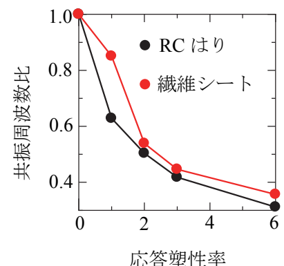
図－4 全体振動試験結果
