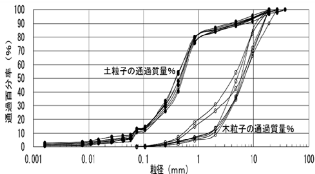
図-4 粒径加積曲線 (No. 5 土粒子・木粒子)
