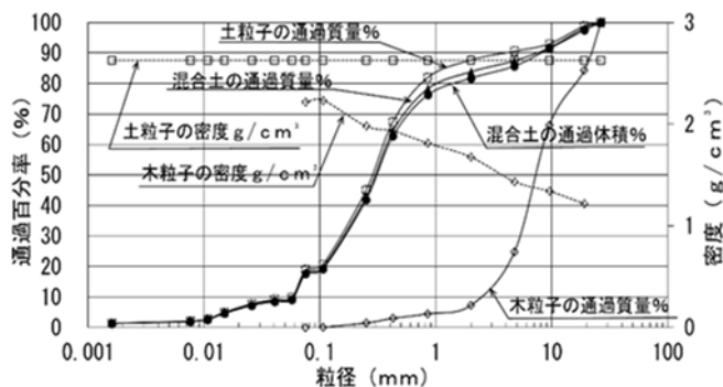
図-3 粒径加積曲線
