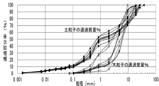
図-5 粒径加積曲線 (No. 6 土粒子・木粒子)
