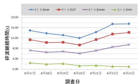
図-7 全砕波継続時間変化
