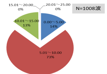
図-5 調査日の全砕波継続時間割合
