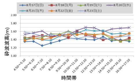
図-4 調査日の砕波波高変化
