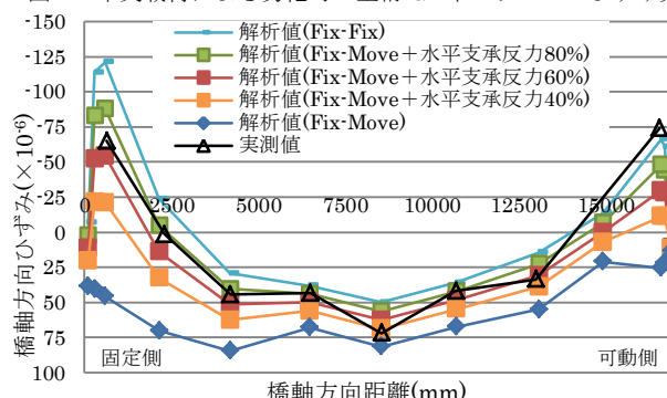
図-5 G2 側偏心載荷による劣化時の主桁 G2 下フランジのひずみ分布
