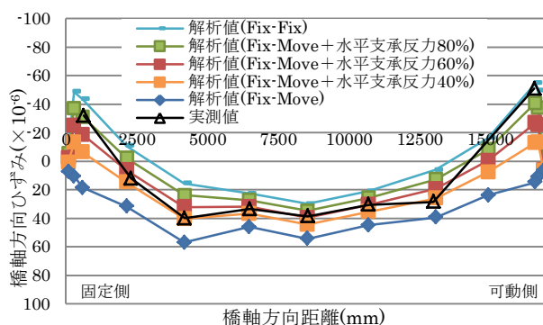
図-3 中央載荷による健全時の主桁 G2 下フランジのひずみ分布
