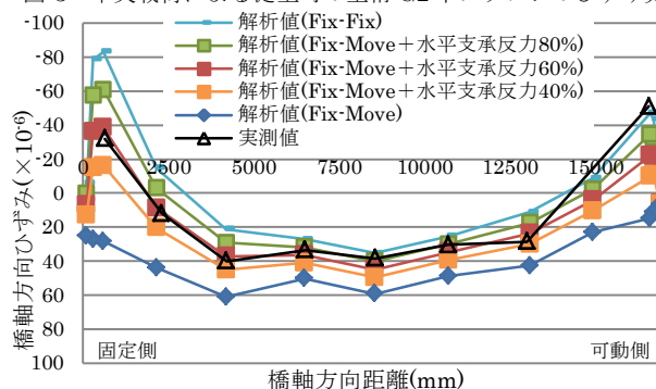
図-4 中央載荷による劣化時の主桁 G2 下フランジのひずみ分布
