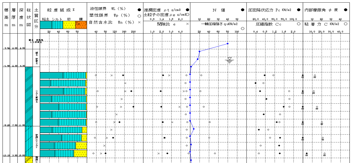
図-1 土性図
