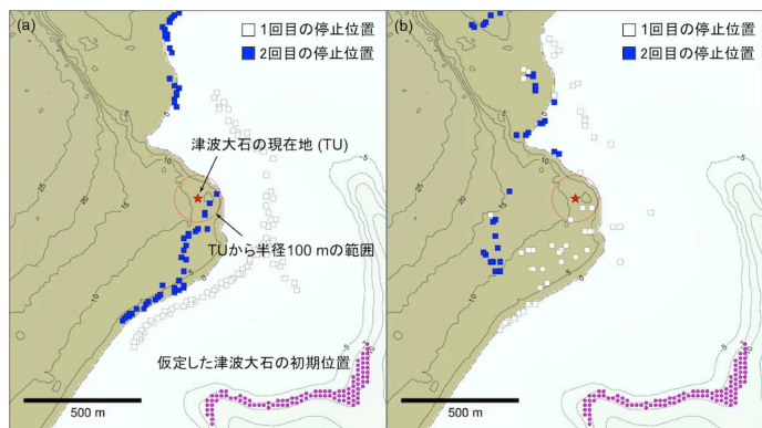
図-2 (a) 津波大石の現在地，仮定した初期位置およびLv. 4 による津波の1回目の停止位置と2回目の停止位置. (b) Lv. 7による津波の1回目の停止位置と2回目の停止位置. モデルを参考に，津波大石の現在地（地点TU）での浸水深が1-8 mになるようなLv. 1-8までの8段階の津波波源モデルを想定し，その組み合わせを消去法によって制約した．なお，巨礫移動数値計算には，Imamura et al. (2008) が提案したBTTモデルを用いた．
