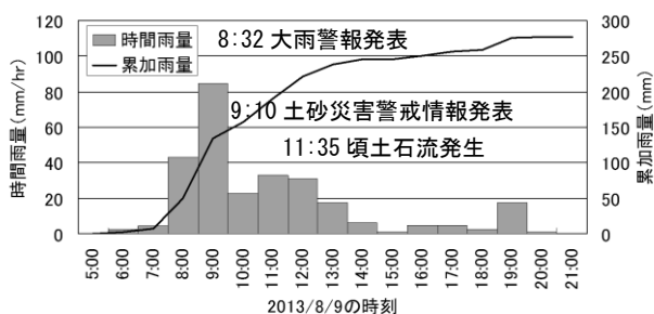
図－1 鎧畑観測所における雨量観測値
