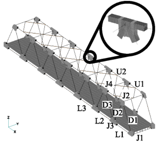
図-1 解析モデルおよび格点部の拡大図
