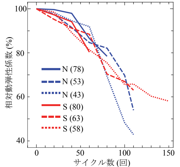
図－2 サイクル数と相対動弾性係数
