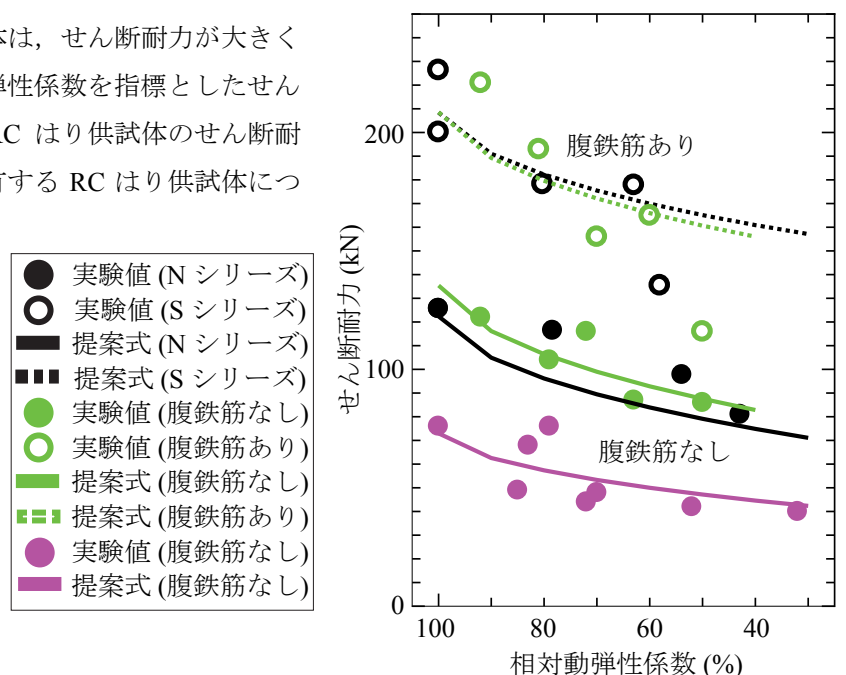
図－4 相対動弾性係数とせん断耐力
