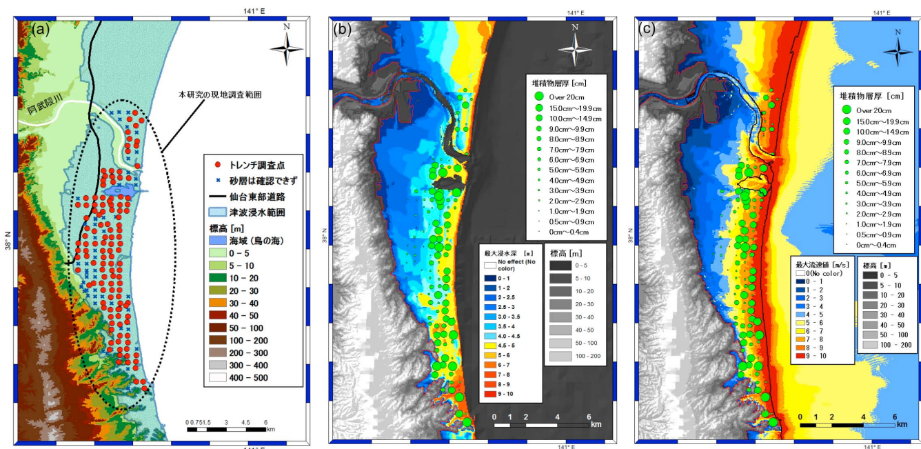
図-1. (a)仙台平野沿岸部の現地調査点．地形は国土地理院公開の震災前10 m DEM，津波浸水範囲は日本情報地理学会公開データを使用．(b)津波堆積物層厚と最大浸水深(計算)の関係．(c)津波堆積物層厚と最大流速(計算)の関係．
