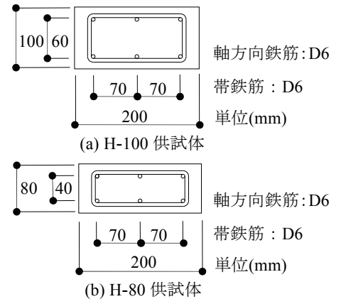
図-2 橋脚模型の断面図
