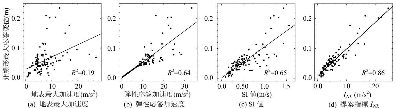
図-1 地震動強度指標と非線形最大応答変位の比較
