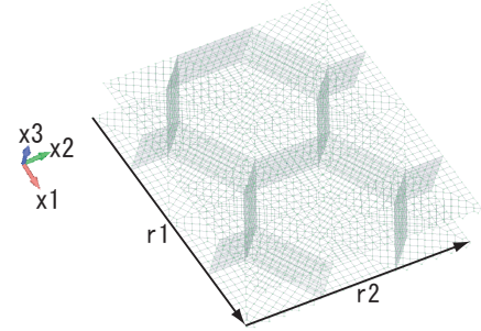
図-1 セル状サンドウィッチパネル
