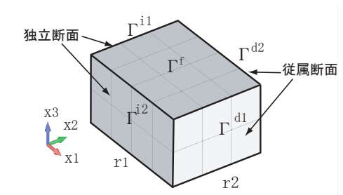
図-1 セル状サンドウィッチパネル
