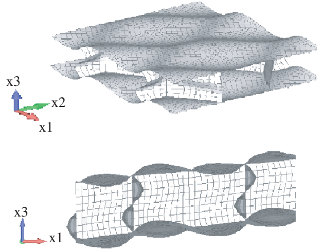
図-3 せん断変形図
