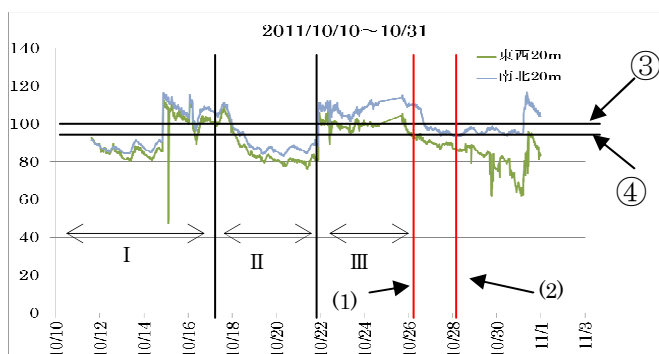
図-6 (1)福島県沖地震 (2)三陸沖地震
