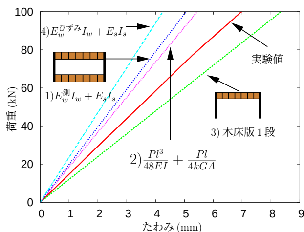
図-5 荷重-たわみグラフ
