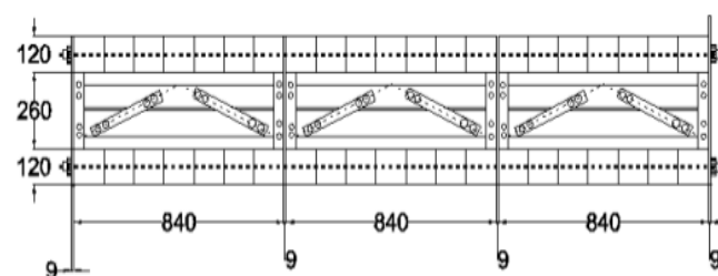
図-1 側面図
