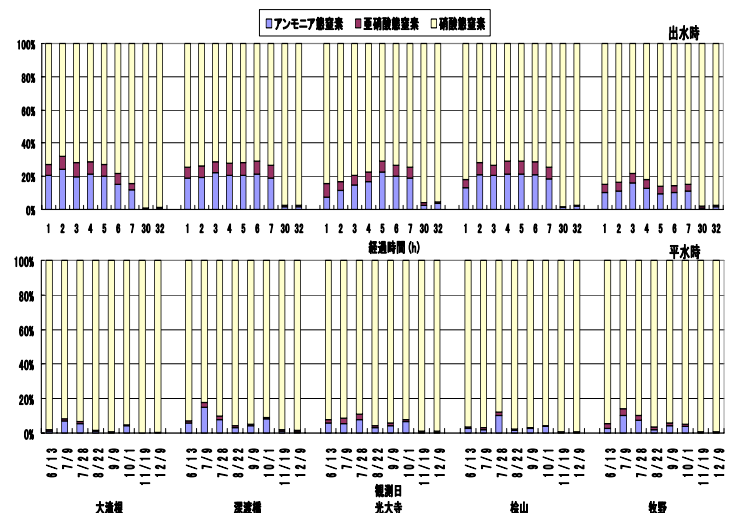
図-7 出水時と平水時の無機三態窒素の割合
