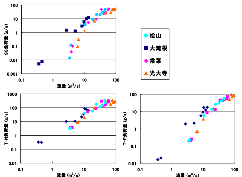
図-6 出水時の各負荷量と流量の関係
