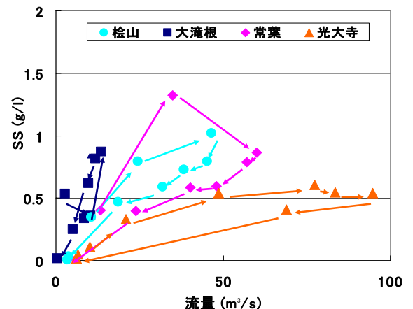
図-3 出水時の SS 濃度と流量の関係
