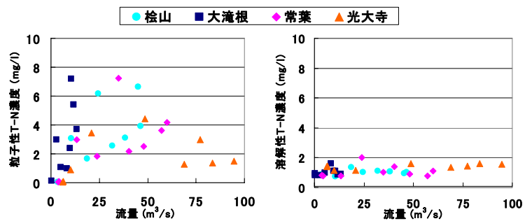
図-4 出水時の粒子性、溶解性 T-N 濃度と流量の関係
