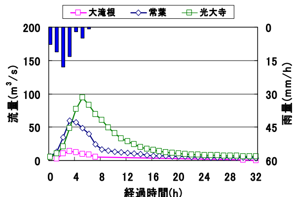
図-2 出水時のハイドロ・ハイトグラフ
