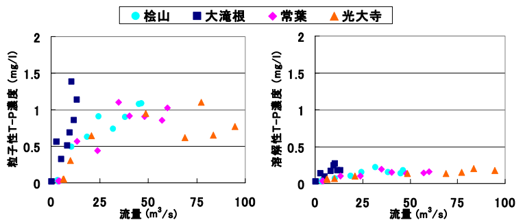
図-5 出水時の粒子性、溶解性 T-P 濃度と流量の関係
