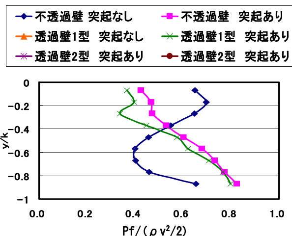
図-4 保護工壁前面に働く圧力の分布特性
