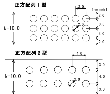
図－2 透過壁形状
