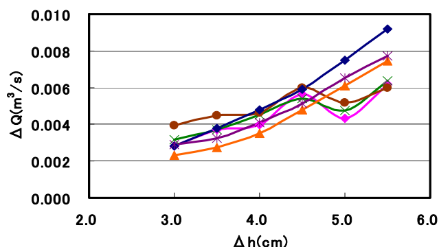
図-5 汜濫流量と越流水深の関係
