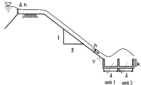
図－1 堤体及び裏法尻保護工
