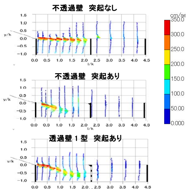
図-3 保護工内の流速ベクトル図
