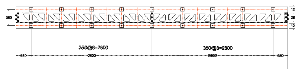
図-3 三角孔を設けた鋼板を用いたモデル
