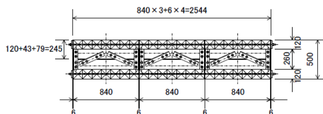
図-1 山形鋼トラスを用いたモデル
