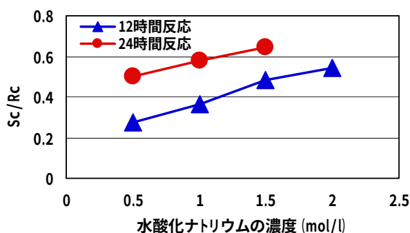
図-4 水酸化ナトリウムの濃度と Sc/Rc の関係
