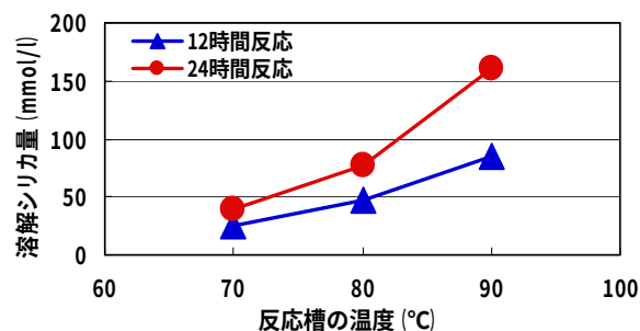
図-1 反応槽の温度と溶解シリカ量 ( Sc ) の関係
