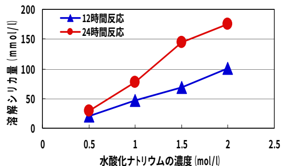
図-3 水酸化ナトリウムの濃度と溶解シリカ量 ( Sc ) の関係
