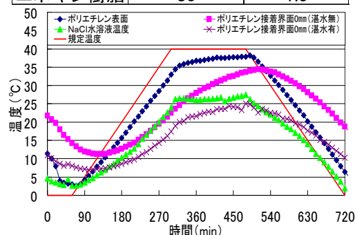
図-1 温度サイクル図 (高温)
