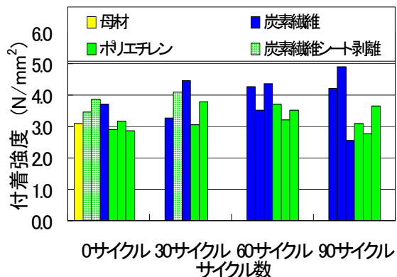
図-5 付着強度試験結果 (低温)
