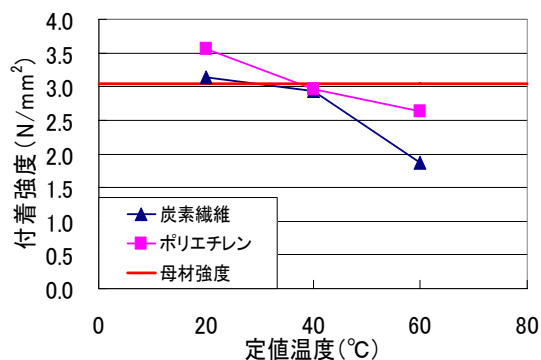
図-7 定値温度による付着強度
