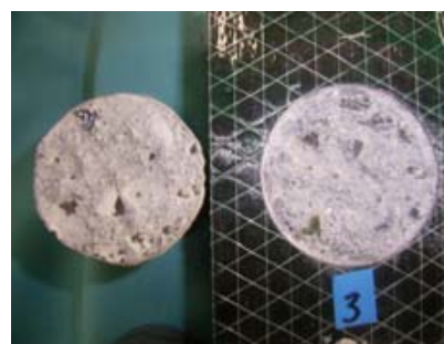
図-6 界面破壊の状況 (炭素繊維)
