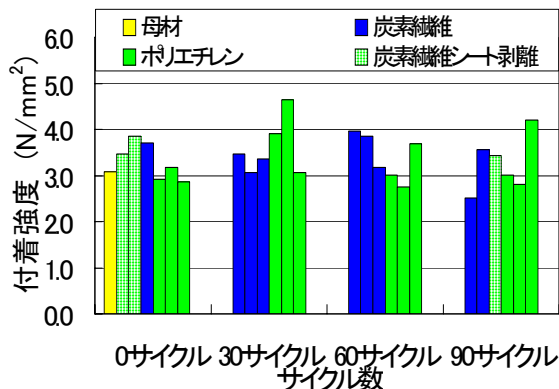
図-4 付着強度試験結果 (高温)
