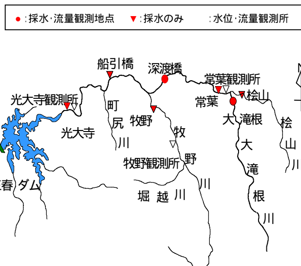
図-1 三春ダム流域平面図
