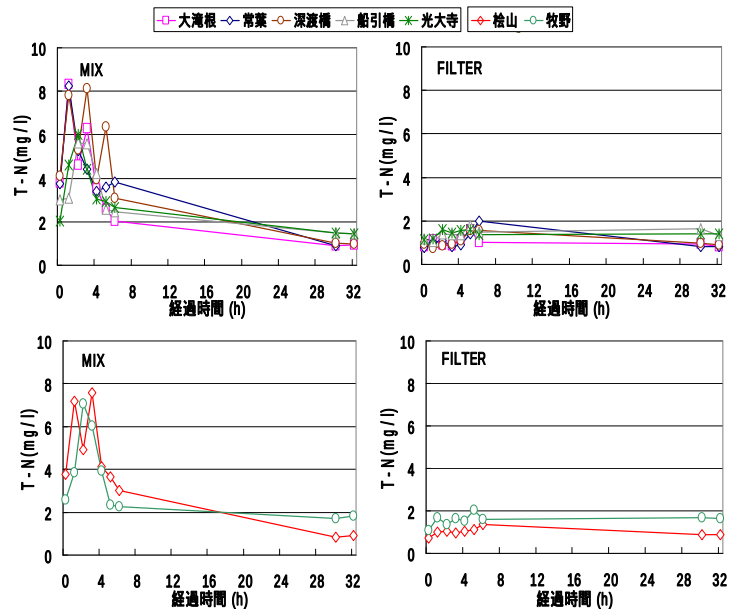
図-4 出水時の総窒素濃度
