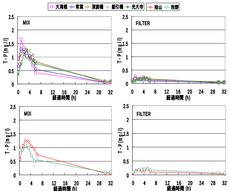
図-5 出水時の総リン濃度
