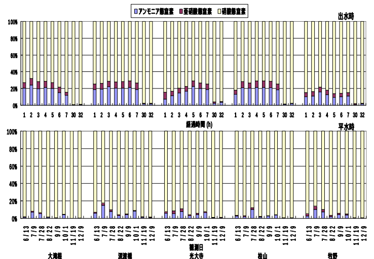
図-6 出水時と平水時の無機三態窒素の割合
