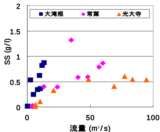
図-3 出水時のSSと流量の関係
