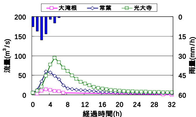
図-2 出水時のハイドロ・ハイトグラフ
