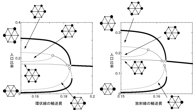
図-4 分岐経路
