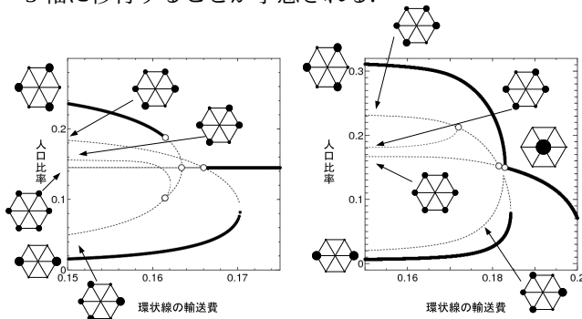
図-2 分岐経路
