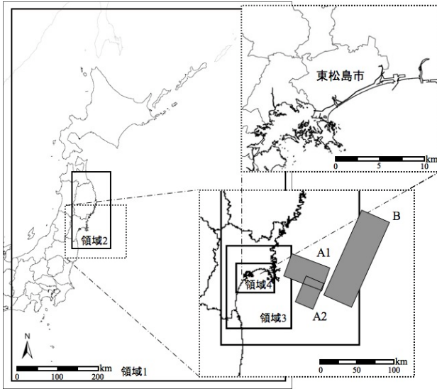
図-1 計算領域及び断層モデル
