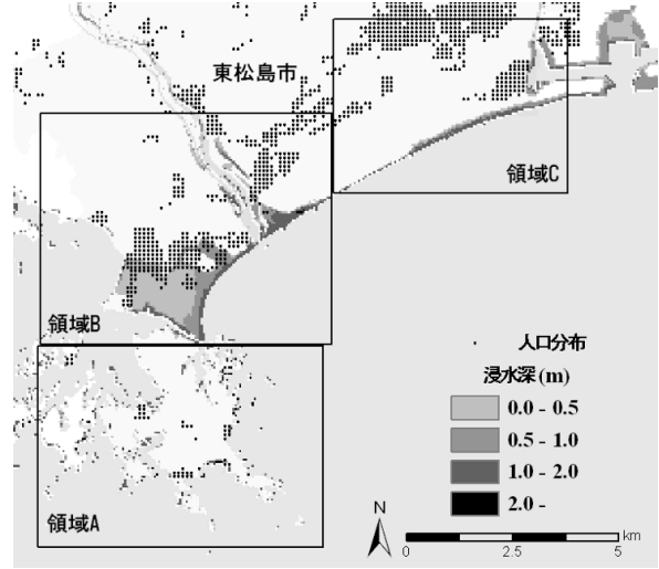
図-2 浸水予測結果
