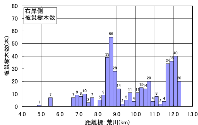
図-3 荒川の被災樹木本数(右岸側)
