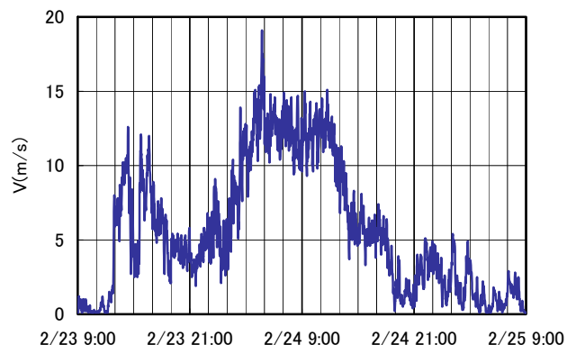
図-1 荒川の風況状況
