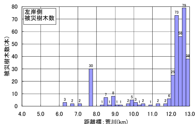
図-2 荒川の被災樹木本数(左岸側)
