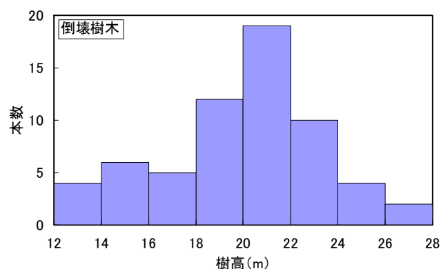
図-3 被災樹木の樹高と本数の関係
