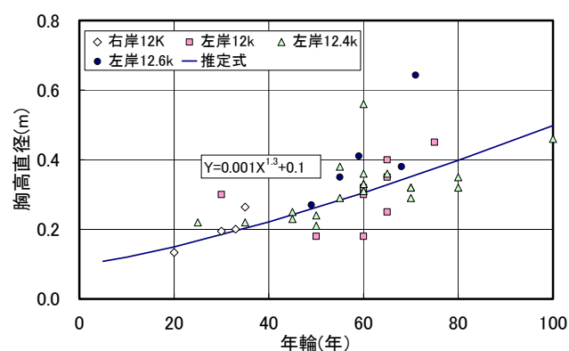
図-4 年輪と胸高直径との関係
