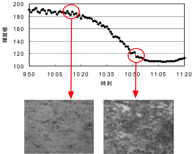
図4 積雪 湿潤の検知
