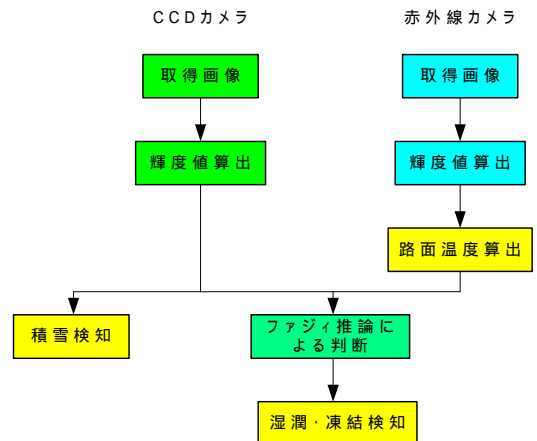
図8 路面状況判別システム
