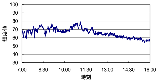
図5 湿潤 凍結の検知
