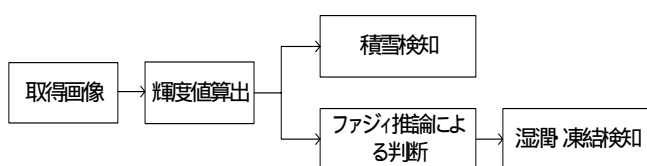
図6 路面状況判別手順
