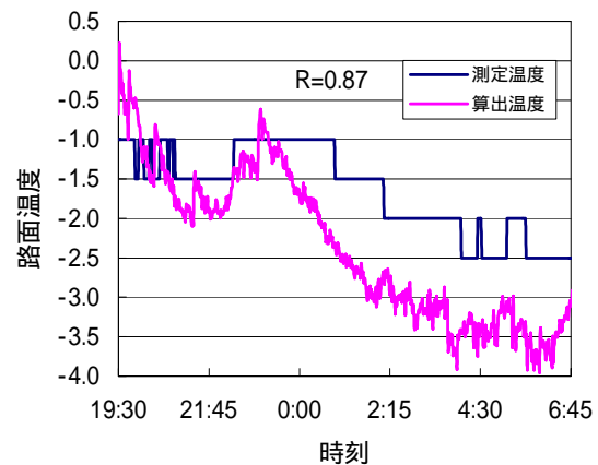
図3 測定路面温度と算出路面温度
