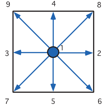
図-1 二次元9速度格子
