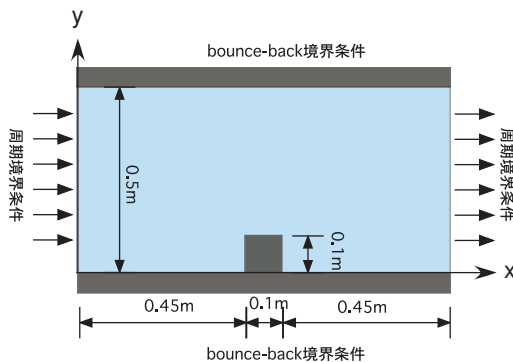
図-2 定義図
