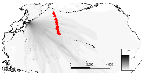
図-2 2003十勝沖地震津波の最大波高分布
