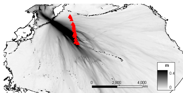
図-1 2006千島列島沖地震津波の最大波高分布
