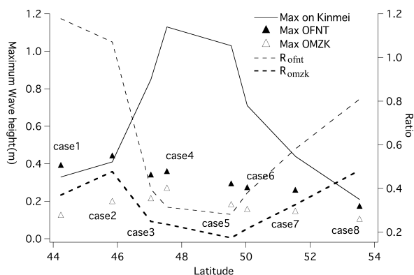
図-4 後続波と欽明海山上での最大波高及び波高比
