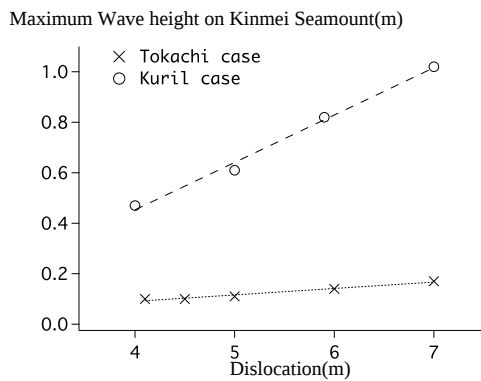
図-3 滑り量の変化に対する欽明海山上での最大波高の変化
