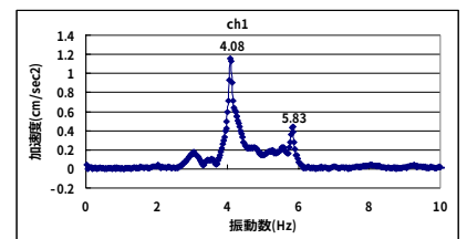
図－5 平成 19 年度 スペクトル図
