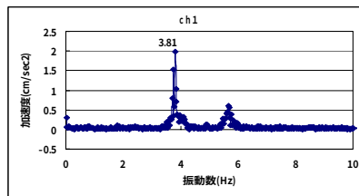
図－2 平成 16 年度 スペクトル図
