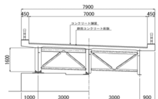
図－1 断面図
