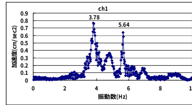
図－4 平成 18 年度 スペクトル図
