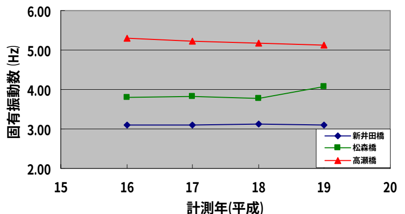
図－6 計測年と固有振動数
