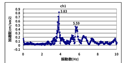
図－3 平成 17 年度 スペクトル図
