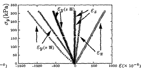
図-5 試験体 (y)
