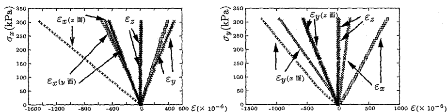
図-4 試験体 (x)
