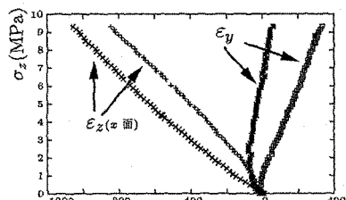
図-7 試験体 (π型試験体 z)
