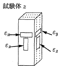
図-2 ひずみゲージ
