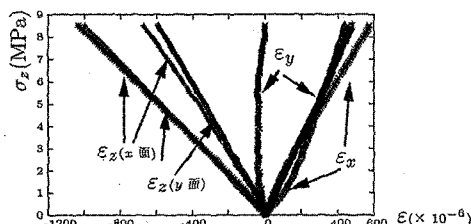
図-6 試験体 (z)
