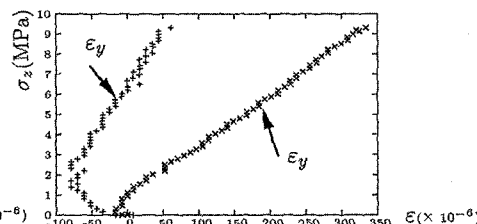
図-8 試験体 (π型試験体 z横)
