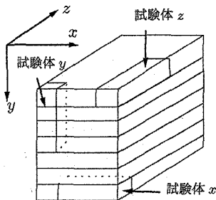
図-1 試験体 x sin z
