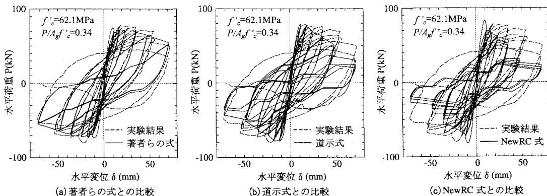
図-2 FHC2-0.34 供試体の荷重－変位関係と解析結果との比較（塑性ヒンジ長 0.5 D(255mm)）
