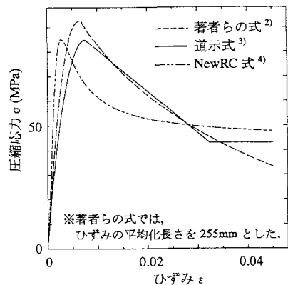
図-1 平均化応力-ひずみ関係の比較
