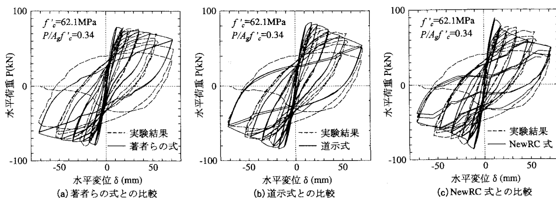
図-3 FHC2-0.34 供試体の荷重－変位関係と解析結果との比較（塑性ヒンジ長 1.0D(510mm)）
