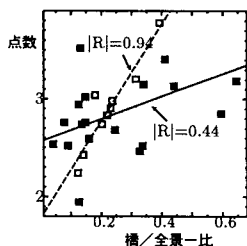
図-10 橋 / 全景 - 比 (白黒)
