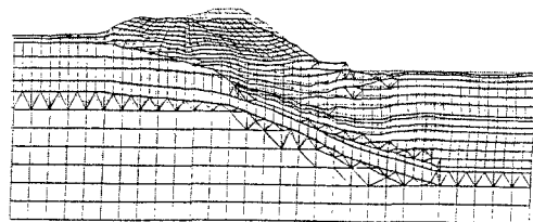
図-6 盛立て解析による初期応力を用いた応答変位 (盛土内最大応答加速度発生時)
