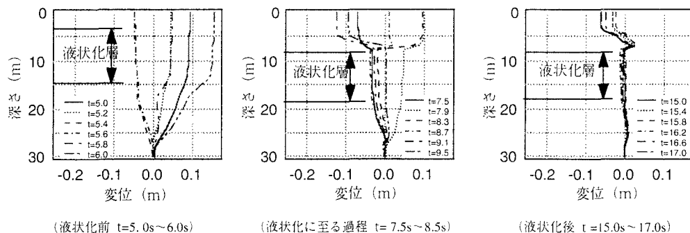
図-5 応答変位の深度分布の経時変化 (ポートアイランドモデル 4)
