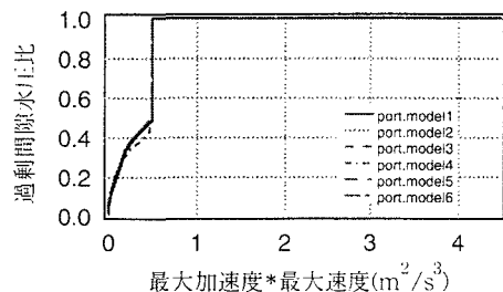
図-6 ポートアイランド入力波に対する最大値指標 と過剰間隙水圧比の関係
