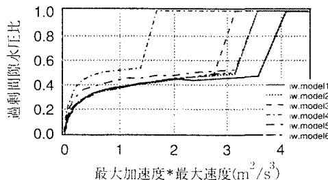
図-7 岩手入力波に対する最大値指標 と過剰間隙水圧比の関係
