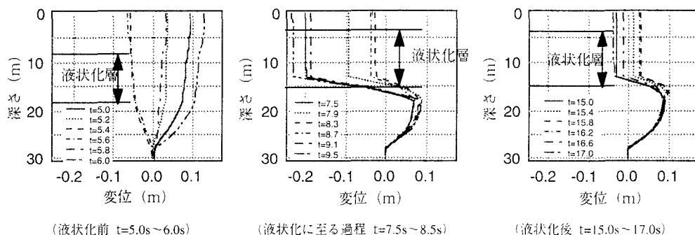
図-4 応答変位の深度分布の経時変化 (ポートアイランドモデル 1)
