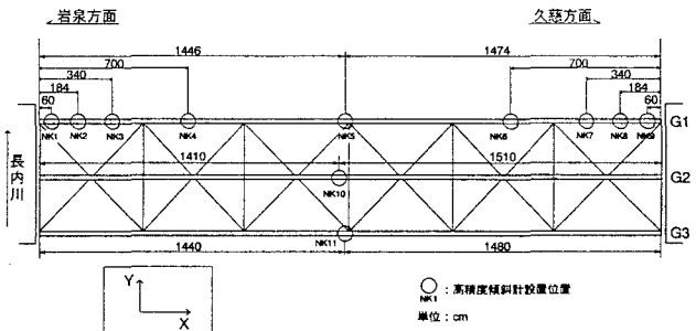
図-1 高精度傾斜計の設置位置
