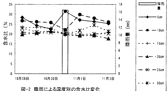
図-2 降雨による深度別の含水比変化
