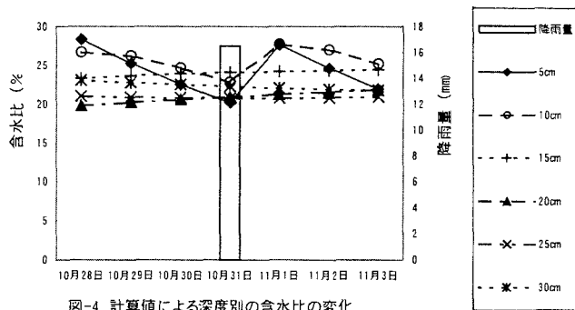
図-4 計算値による深度別の含水比の変化
