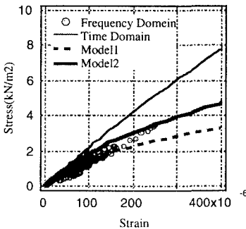
図-5 両手法による低減係数に基づく周波数領域と時間領域における応力-ひずみ関係の比較
