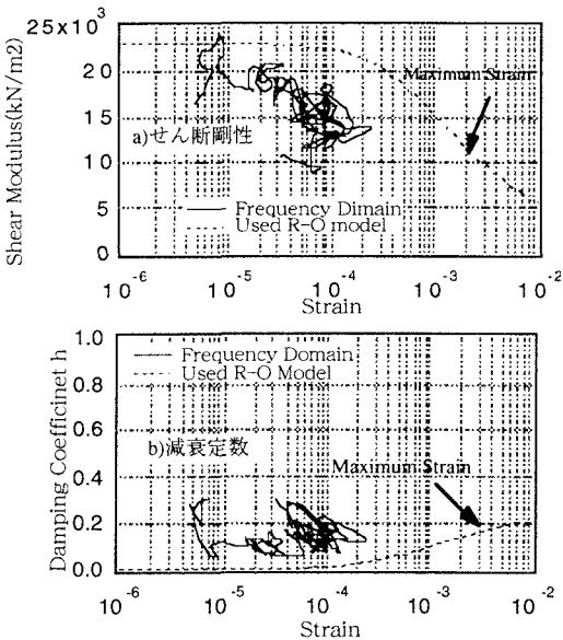
図-2 周波数領域でのせん断剛性及び減衰定数のひずみ依存特性と解析に用いたROモデルの特性の比較
