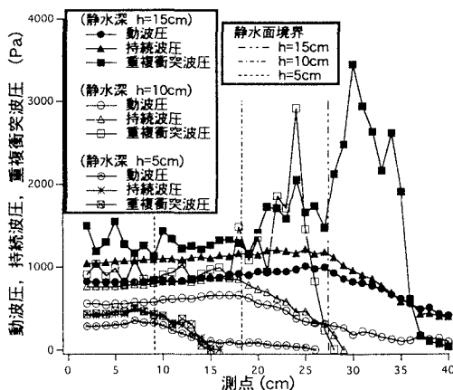
図-4 波圧の測点ごとの変化
