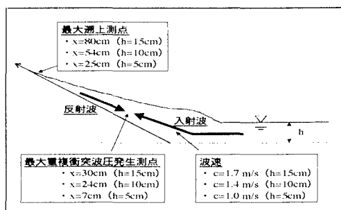
図-5 波速および最大遡上測点
