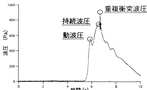
図-2 波圧の時間的変化
