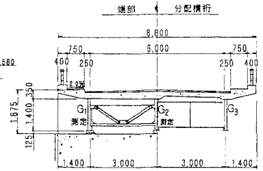
図-2 断面図
