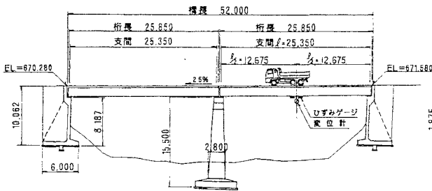
図-1 正徳橋縦断面図
