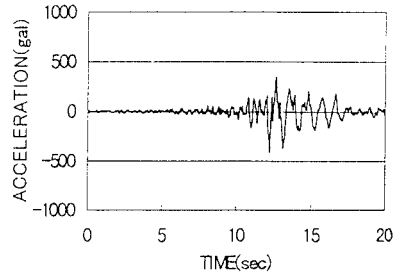
図-5 三陸はるか沖地震波
