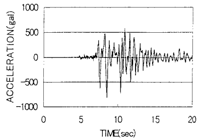
図-4 兵庫県南部地震波
