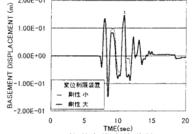
図-6 基礎変位応答曲線
