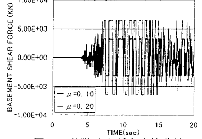
図-8 基礎せん断力応答曲線
