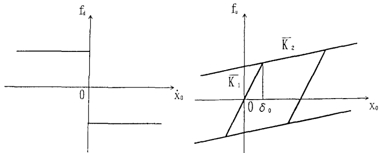
図-2 免震装置の速度・摩擦係関係 図-3 変位制限装置の変位・反力関係
