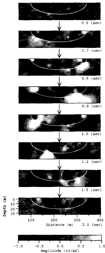
図 5 ひずみ \epsilon_{xx} の応答
