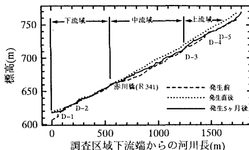
図-2 縦断形状
