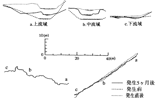
図-4 河道の横断図
