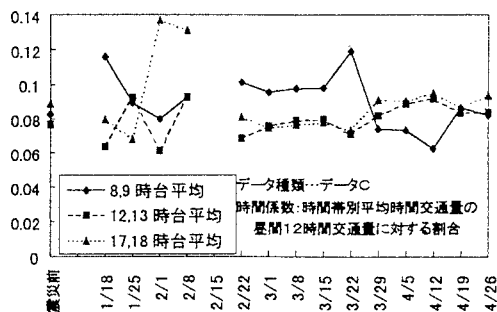
図3 武庫川断面R2下り 時間係数の推移
