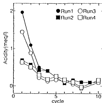
Fig. 4 各cycle最終日(4日目)のpH8.4酸度
