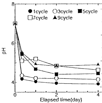
Fig. 2 各cycleのpHの経日変化(Run1)
