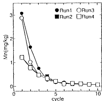
Fig. 7 各cycle最終日(4日目)のMnの溶出量
