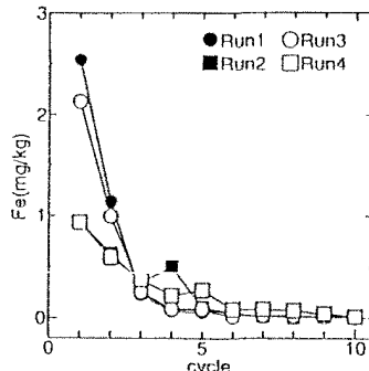
Fig. 6 各cycle最終日(4日目)のFeの溶出量
