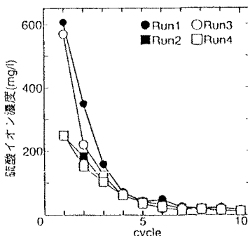
Fig. 5 各cycle最終日(4日目)の硫酸イオン濃度
