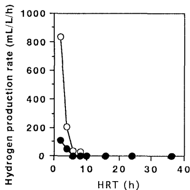
図-3 水素生成速度
