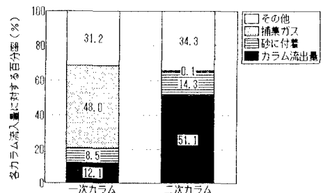
図-8 CODcr収支
