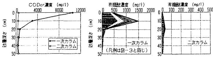
図-4 砂層内でのCODcrと有機酸濃度の変化(71週)
