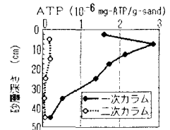
図-6 ATPの変化
