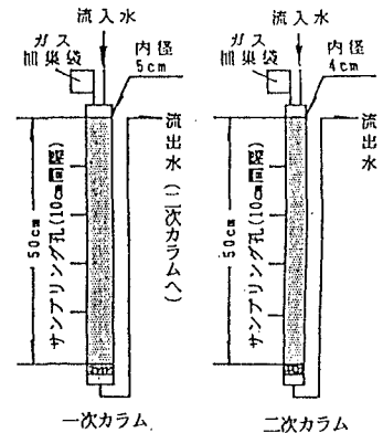
図-1 実験装置
