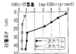
図-5 CODcr付着量の変化
