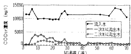
図-2 CODcr濃度の変化
