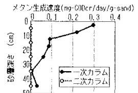
図-7 メタン生成速度の変化
