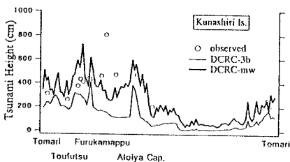
図-3 津波打ち上げ高比較
