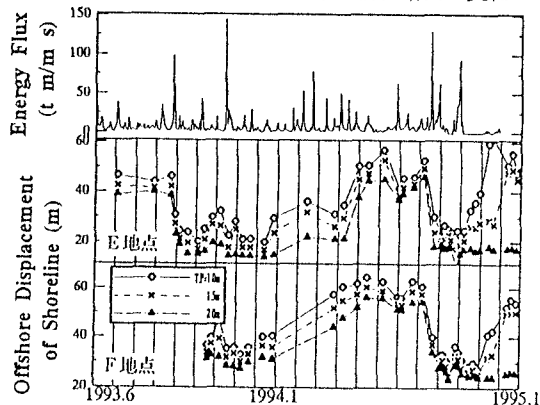
図3. エネルギーフラックスと汀線変動
