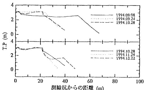
図2. F地点における前浜断面の変化
