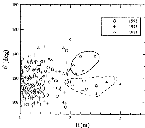
図5. 波高-波向角度 関係
