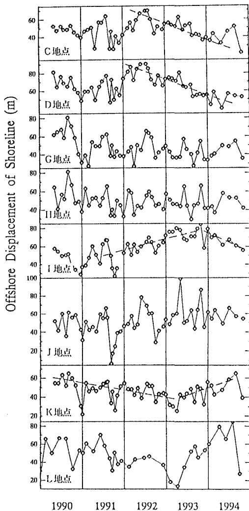
図4. 仙台港南部の汀線変動
