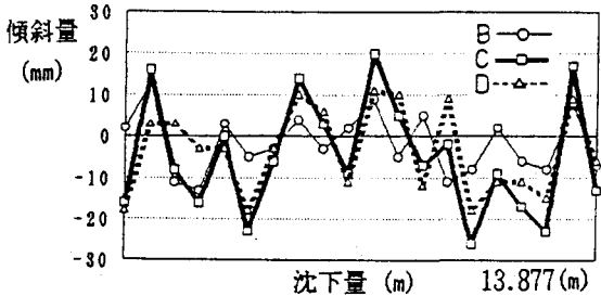
図-2 P4ケーソン傾斜量計測結果
