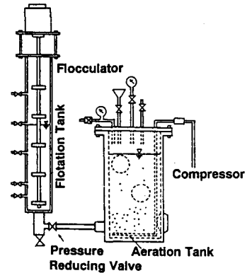
図-1 フローテーションスター
