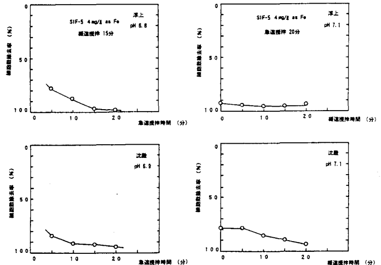
図-2 a 急速攪拌時間の影響
