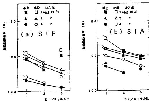
図-5 a, b Si/Metalモル比の影響
